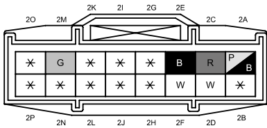
0920-201B AUDIO UNIT
